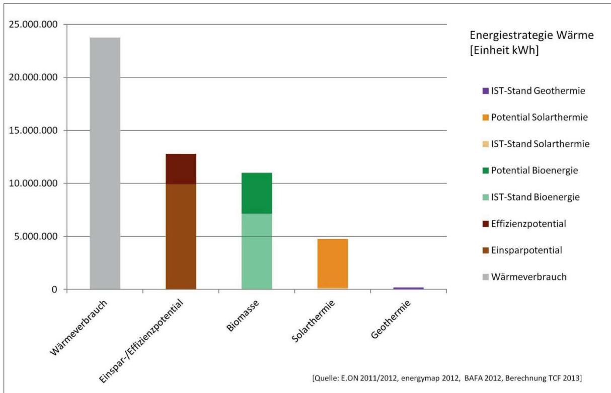
Abbildung C: Energiestrategie Wärme Langdorf
