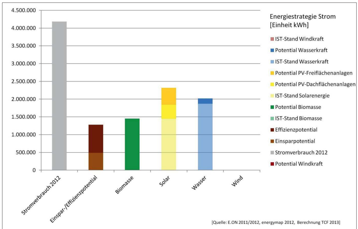
Abbildung D: Energiestrategie Strom Langdorf
