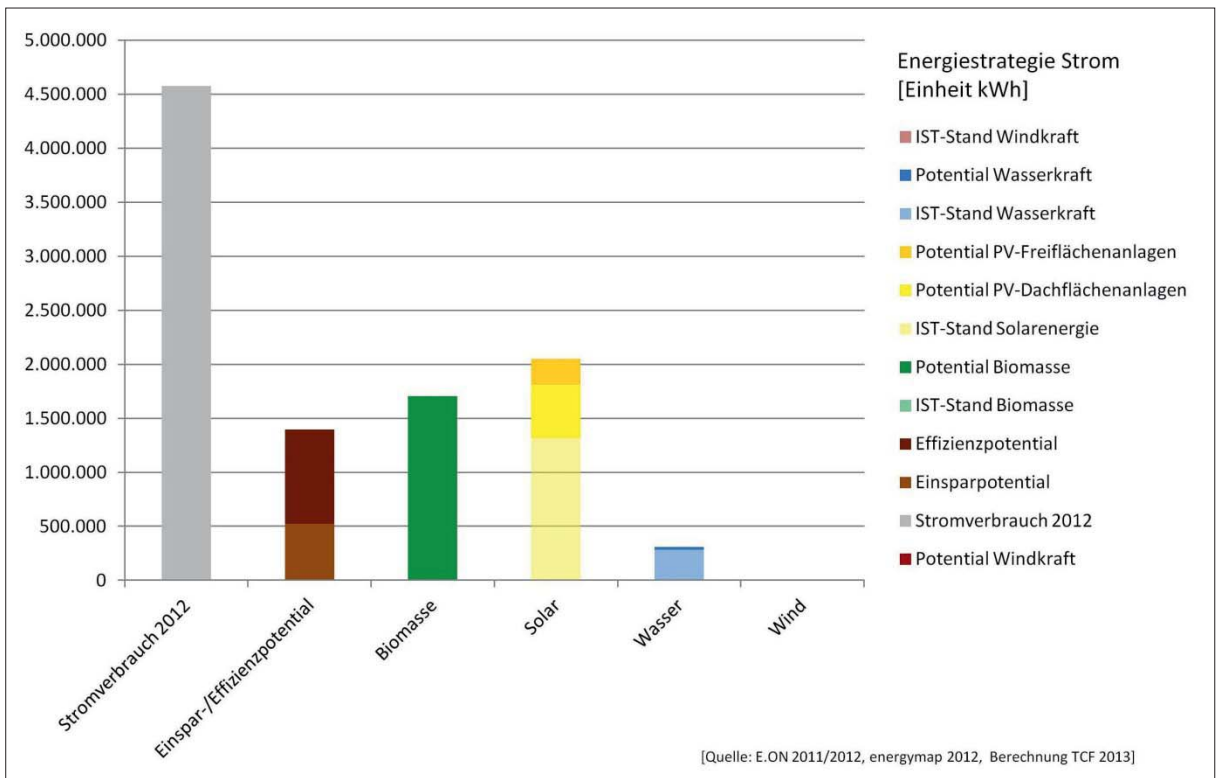
Abbildung D: Energiestrategie Strom Patersdorf
