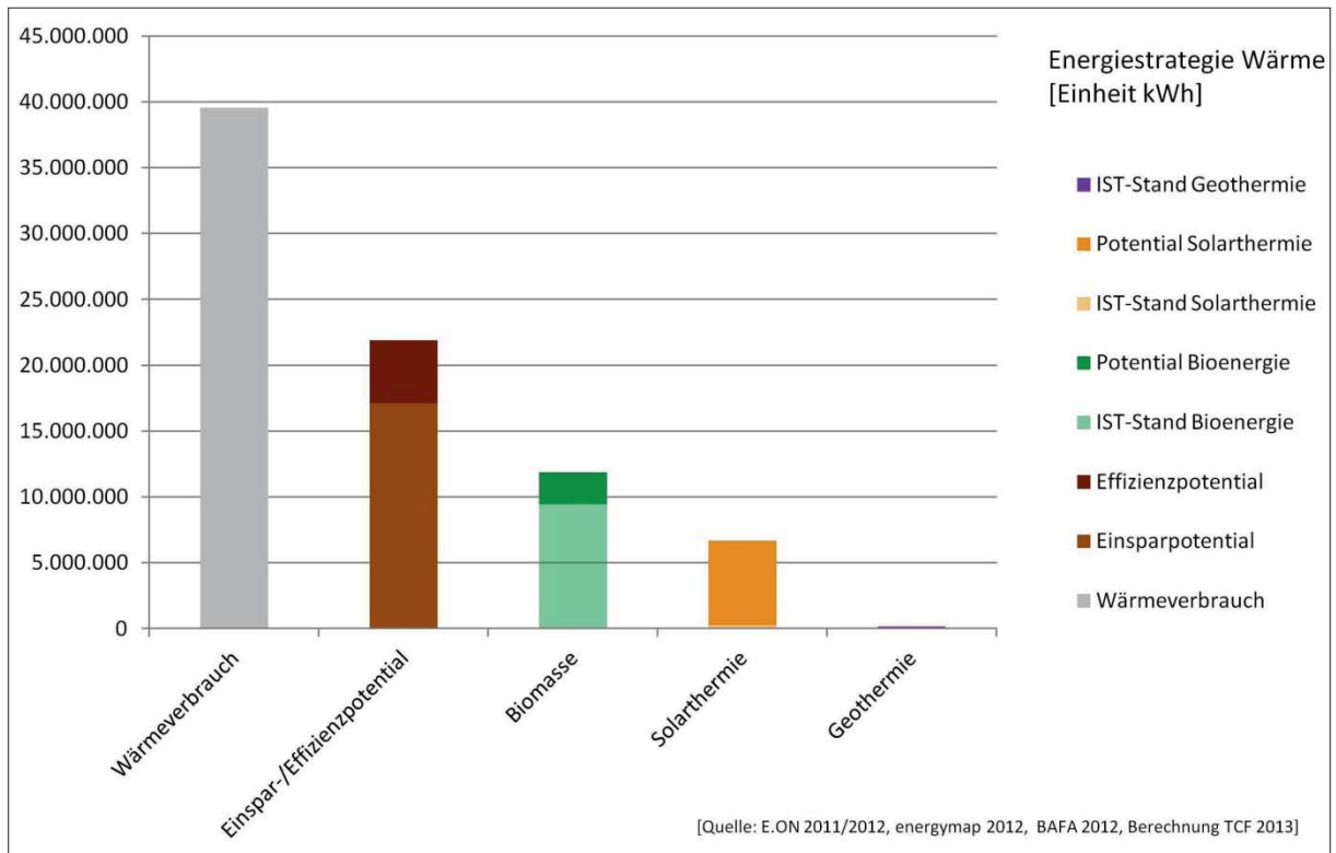
Abbildung C: Energiesstrategie Wärme Prackebach
