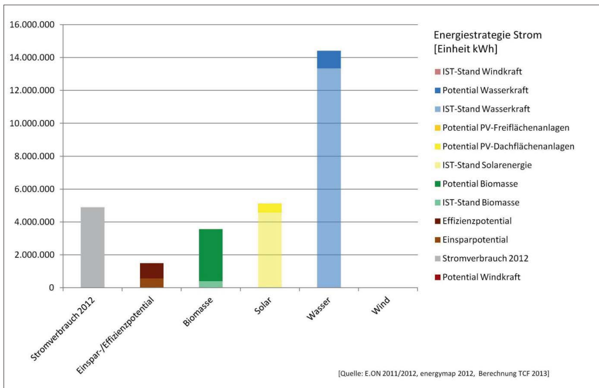
Abbildung D: Energiesstrategie Strom Prackebach
