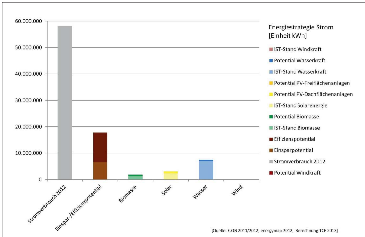
Abbildung D: Energiestrategie Strom Teisnach
