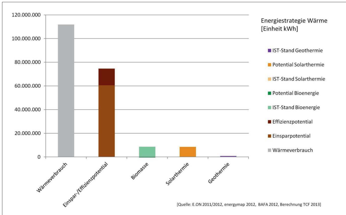
Abbildung C: Energiestrategie Wärme Teisnach
