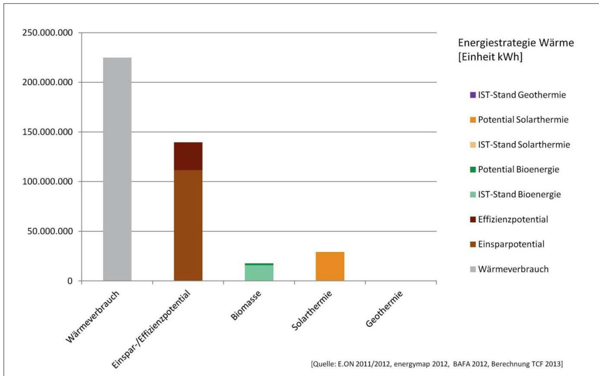
Abbildung C: Energiesstrategie Wärme Viechtach
