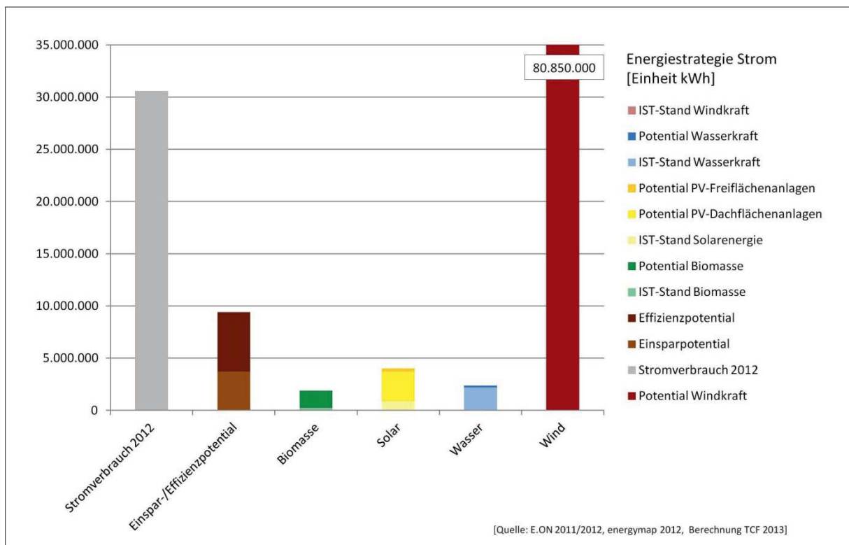
Abbildung D: Energiestrategie Strom Zwiesel
