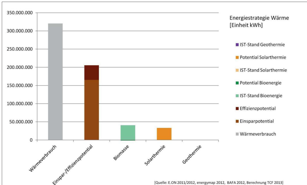
Abbildung C: Energiestrategie Wärme Zwiesel
